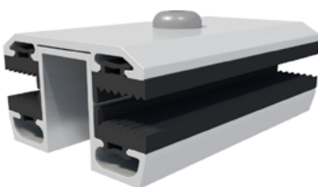
Laminatmittelklemme (LMK)
